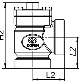
承插焊图示 SOC
