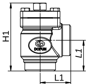
对接焊图示 BW
